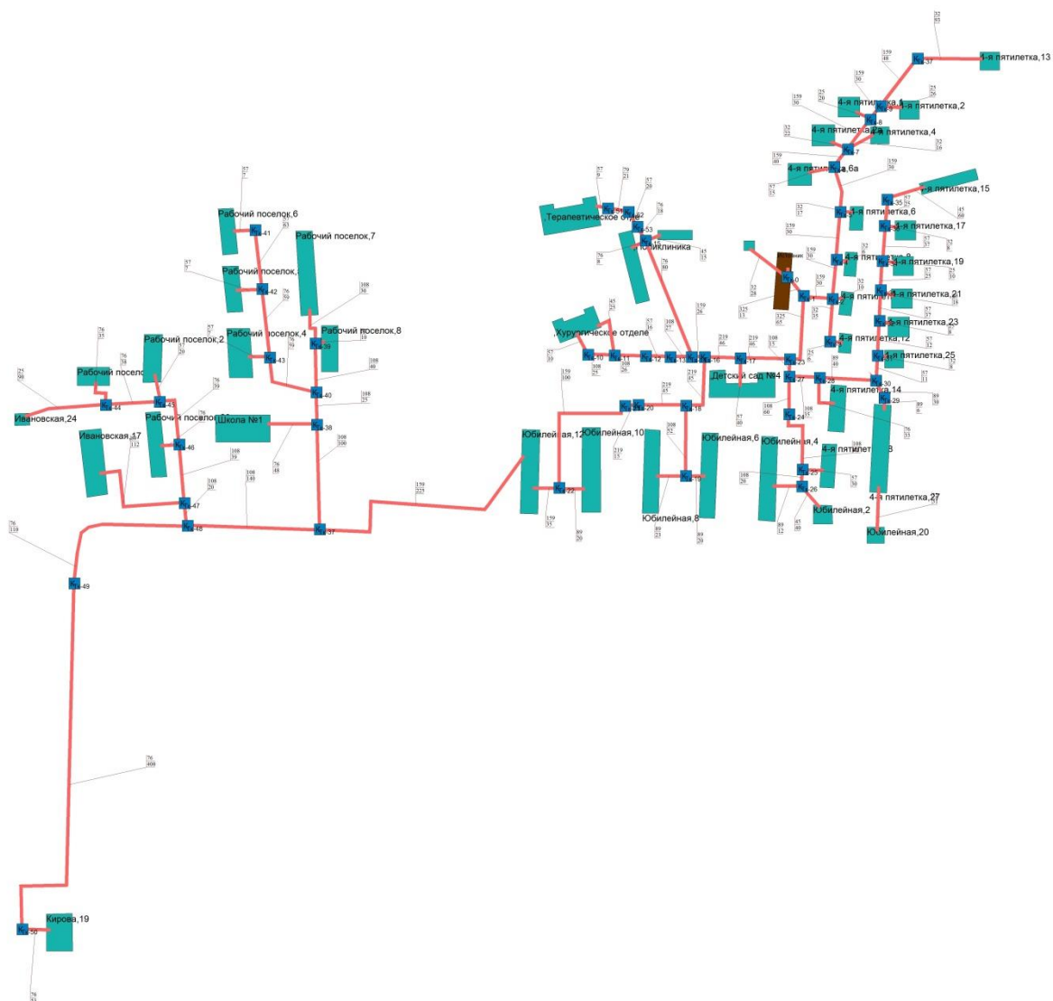
Рисунок 2 - Расположение источника тепловой энергии котельной Квартала А.
